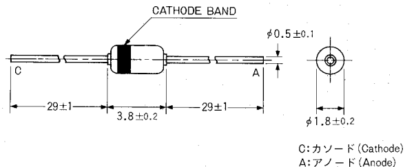
図1 JEDEC: DO-35 EIAJ: SC-40
